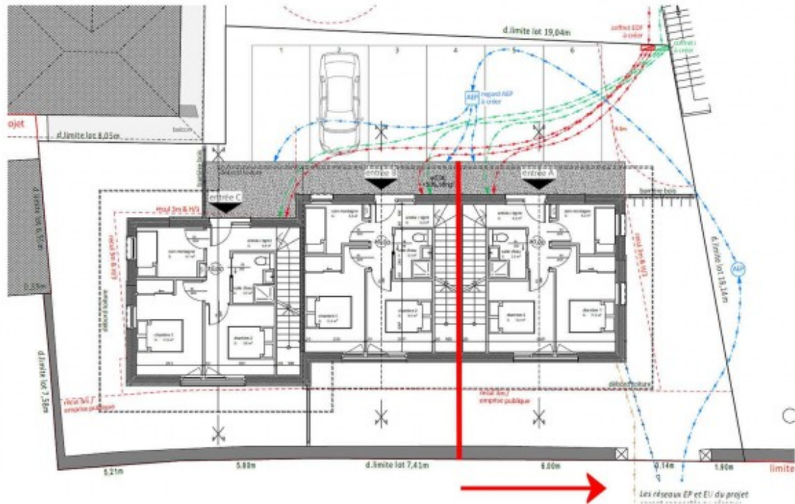
plan rez de jardin
