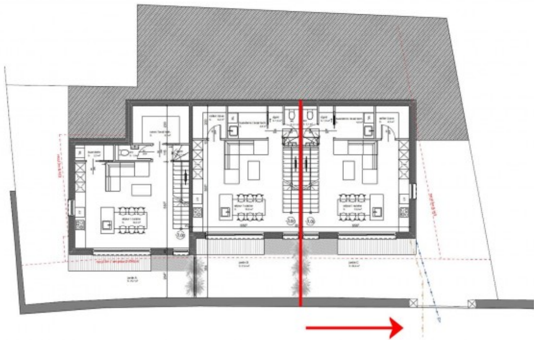
plan rez de jardin
