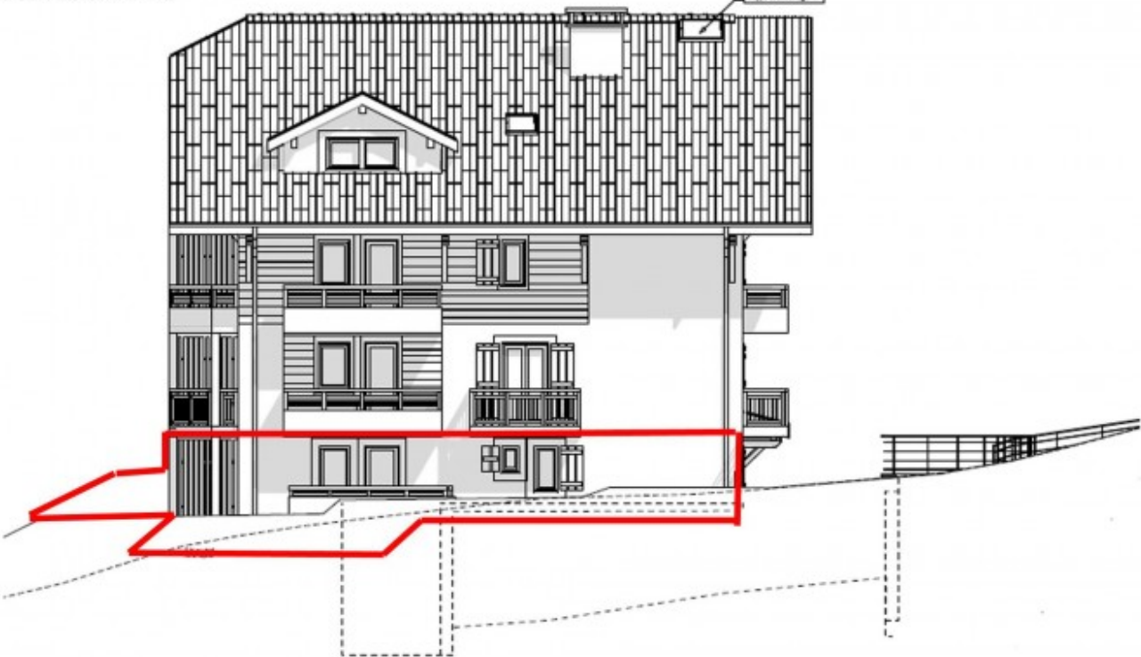
Facade Nord
